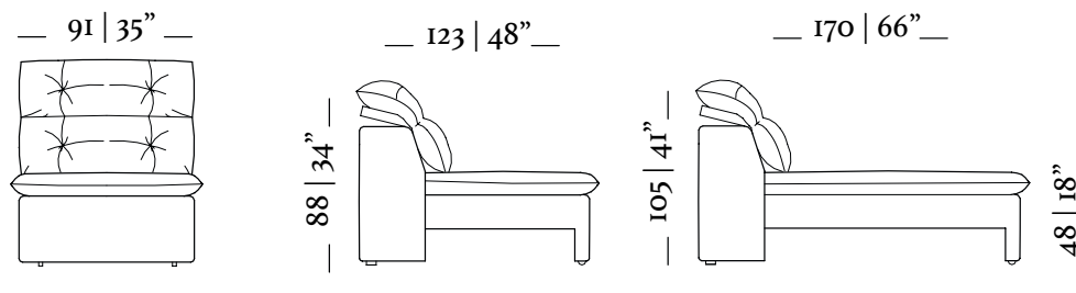
Chaise retrátil/ Retractable chaise sem braços/ no arms Ass. 90cm
