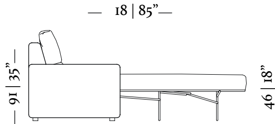
Sofá cama/ Sofa bed 1 Braço reto/ Straight arm
