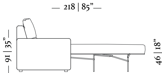
Sofá cama/ Sofa bed Sem braços/ No arms
