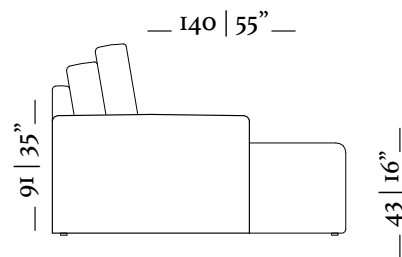
Chaise retrátil/ retractable chaise 2 Braços/ arms 18cm Ass. 80cm
