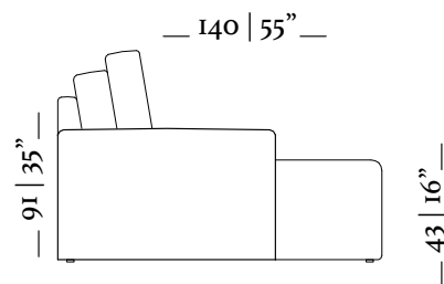
Chaise retrátil/ retractable chaise 2 Braços/ arms 18cm Ass. 70cm
