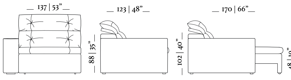
Chaise retrátil/ Retractable chaise 1 braço/ arm 25cm Ass. 110cm
