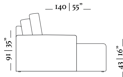
Chaise retrátil/ retractable chaise 2 Braços/ arms 25cm Ass. 70cm
