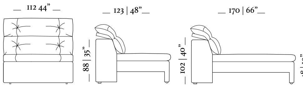
Chaise retrátil/ Retractable chaise Sem braços/ No arm Ass. 110cm
