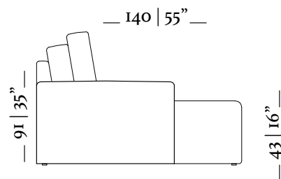
Chaise retrátil/ retractable chaise 2 Braços/ arms 12cm Ass. 110cm
