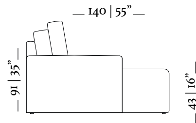
Chaise retrátil/ retractable chaise 2 Braços/ arms 12cm Ass. 70cm
