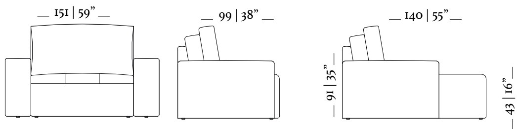
Chaise retrátil/ retractable chaise 2 Braços/ arms 25cm Ass. 100cm
