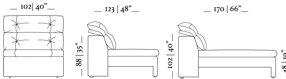
Chaise retrátil/ Retractable chaise Sem braços/ no arms Ass. 100cm
