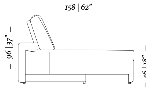
Chaise retrátil/ retractable chaise Sem braços/ no arms Ass. 90cm
