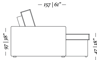
Chaise retrátil/ Retractable chaise 1 Braço/ Arm 18cm Ass. 100cm
