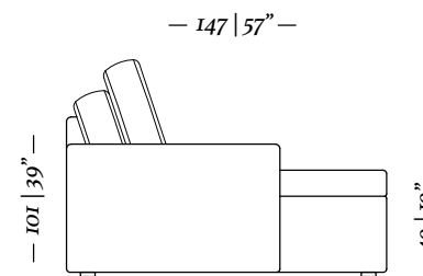
Chaise retrátil 2 Lugares com 2 braços 199 x 103 x 101
