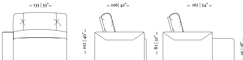
Chaise retrátil 01 Braço, Ass. 110 133 x 106 x 102cm
