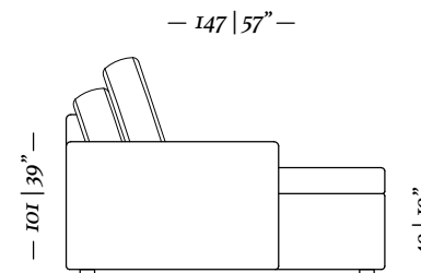
Chaise retrátil 2 Lugares com 1 braço 180 x 103 x 101
