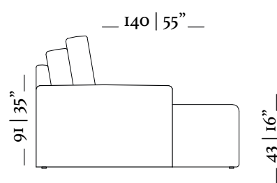
Chaise retrátil/ retractable chaise 2 Braços/ arms 25cm Ass. 90cm
